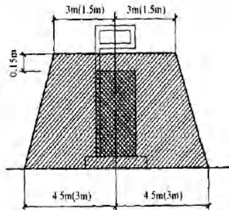
图 3.2-2 汽油加油机操作危险区域划分图
