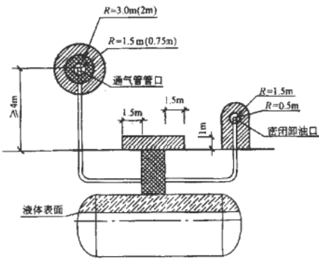
图 3.2-1 埋地卧式汽油储罐爆炸危险区域划分图 图 3.2-2 汽油加油机操作危险区域划分图
