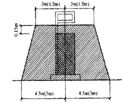
图 3.2-2 汽油加油机操作危险区域划分图
