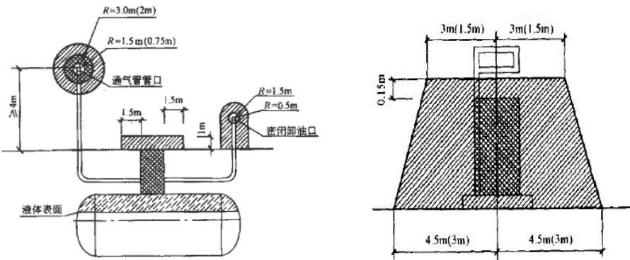
图 3.2-1 埋地卧式汽油储罐爆炸危险区域划分图 图 3.2-2 汽油加油机操作危险区域划分图
