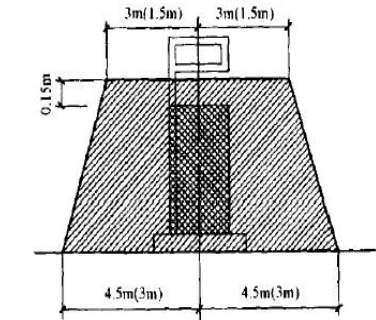
图 3.2-2 汽油加油机操作危险区域划分图
