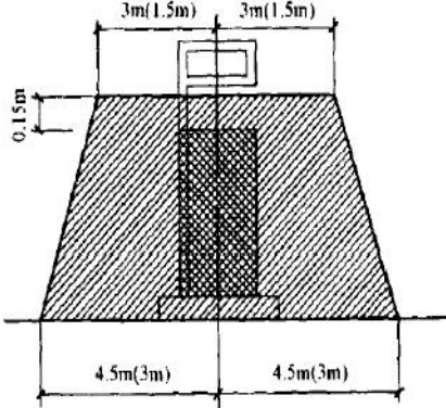
图 3.2-2 汽油加油机操作危险区域划分图
