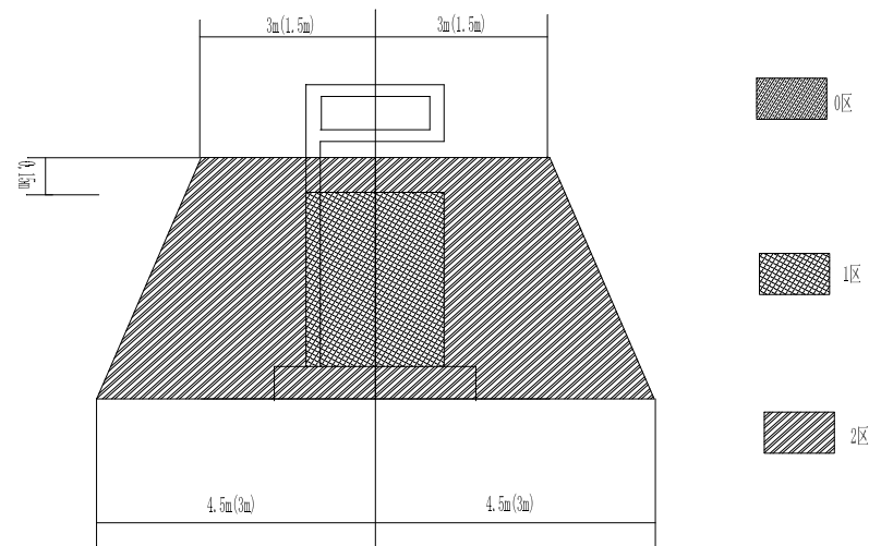
图 3-1 加油机爆炸危险区域划分
