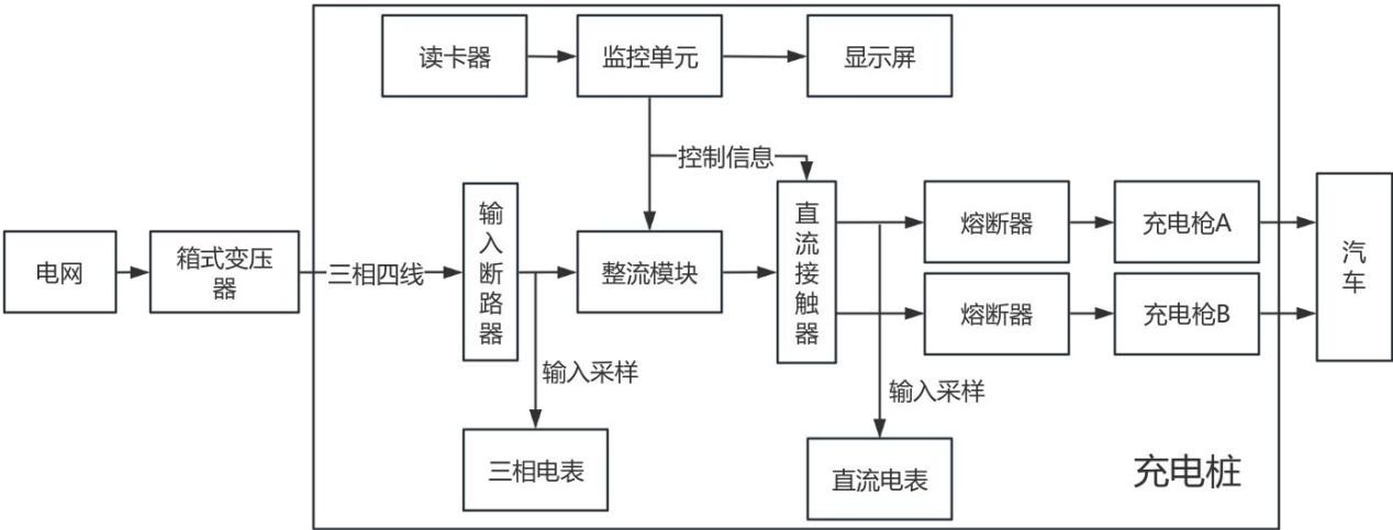
图 1-7 充电工艺流程示意图
