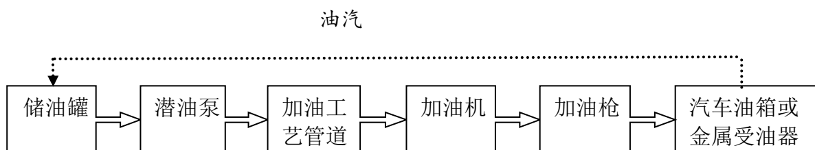
图 1-4 汽油加油工艺流程
