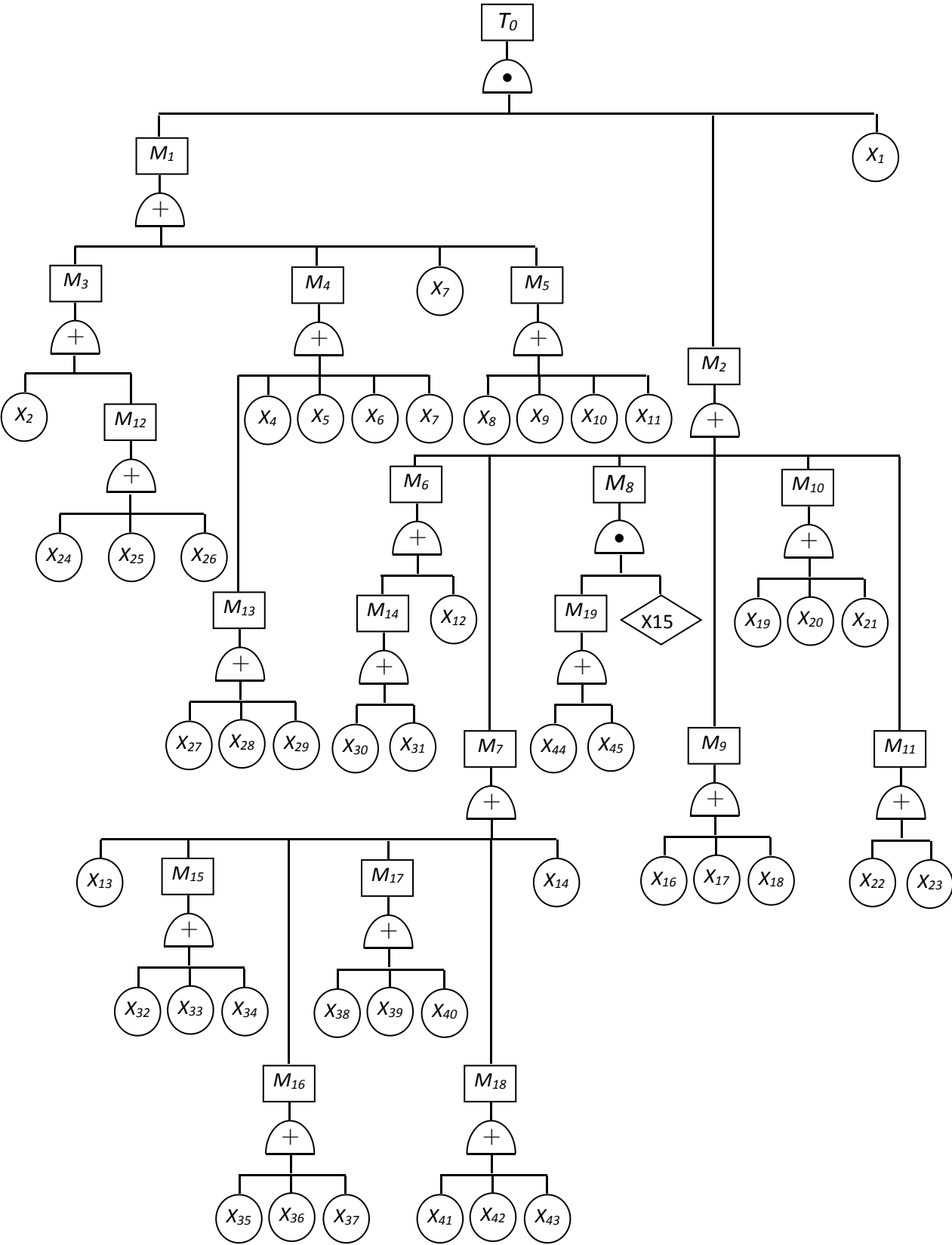
图 2-4 事故树分析
