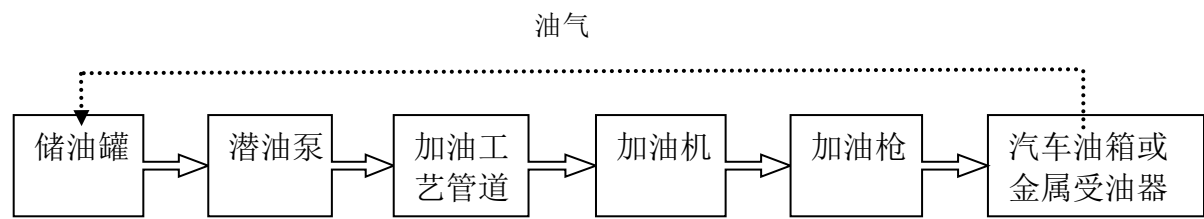
图 2-5 汽油加油工艺框图
