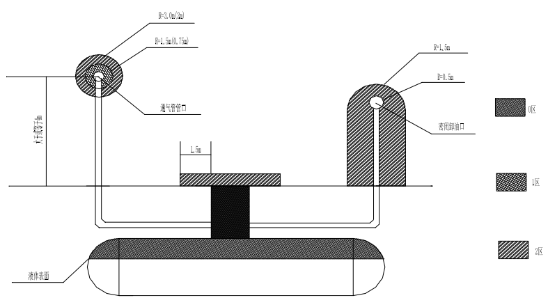
图 3-2 油罐车卸油爆炸危险区域划分
