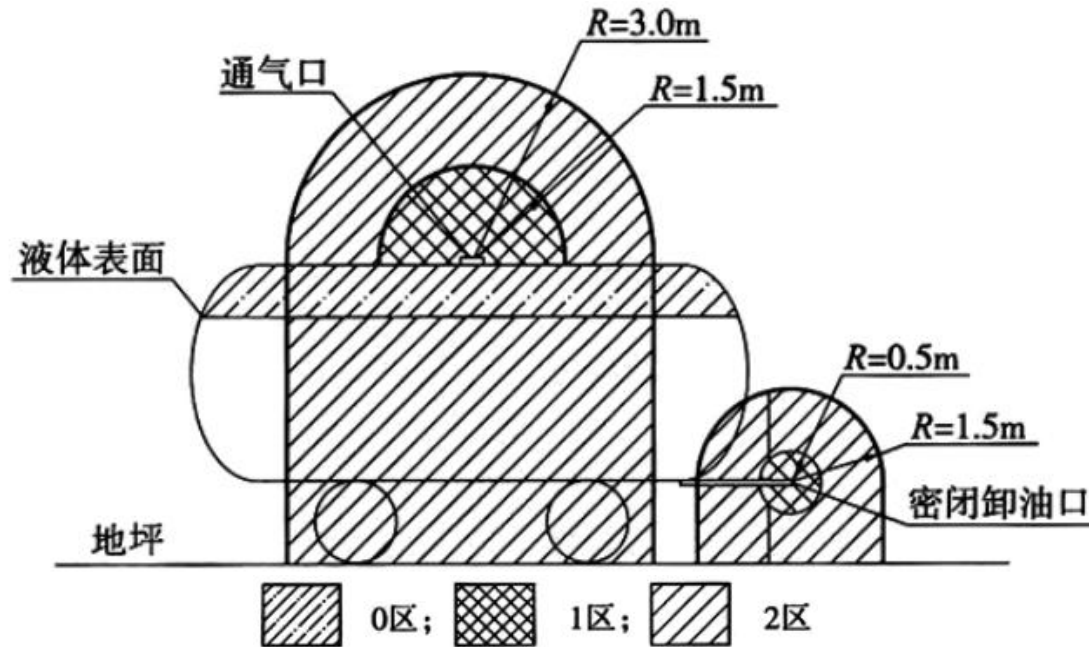
图 3-3 汽油埋地油罐爆炸危险区域划分
