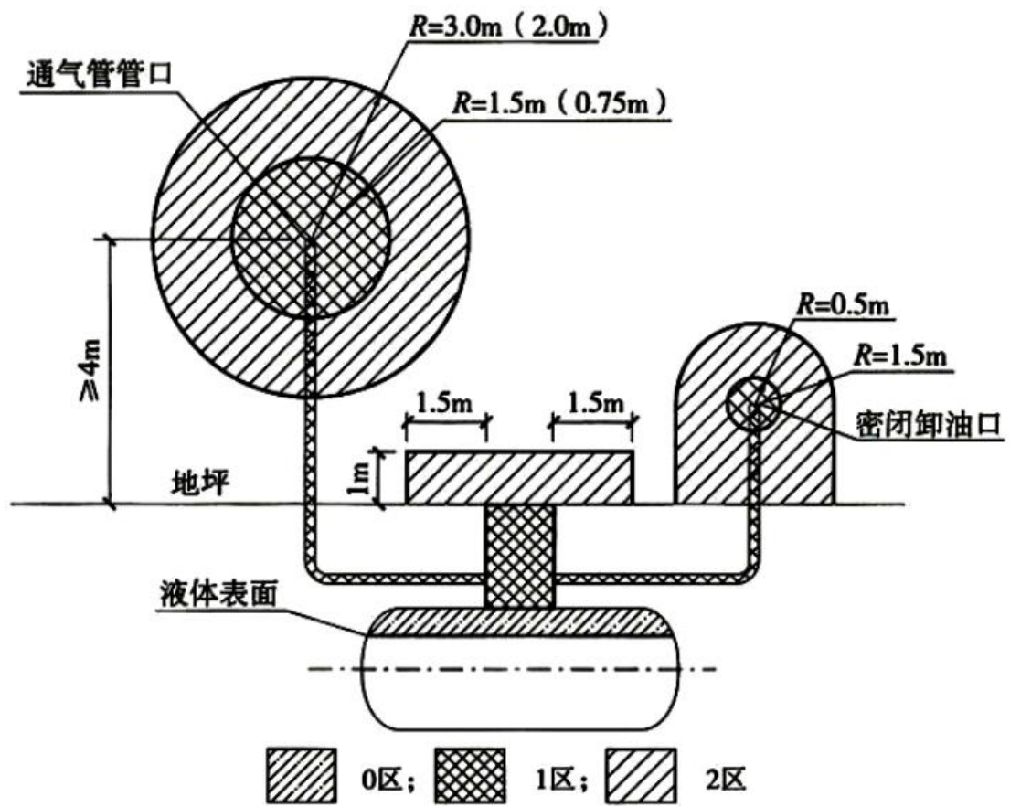
图 3-2 汽油油罐车卸油爆炸危险区域划分
