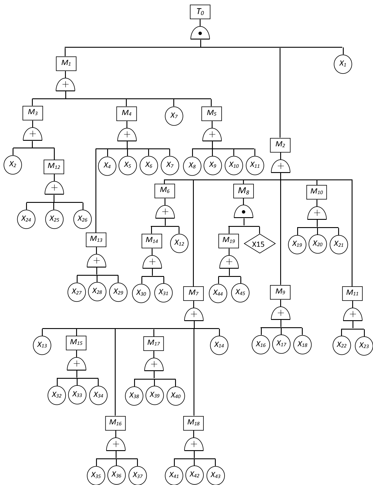
图 2-4 事故树分析
