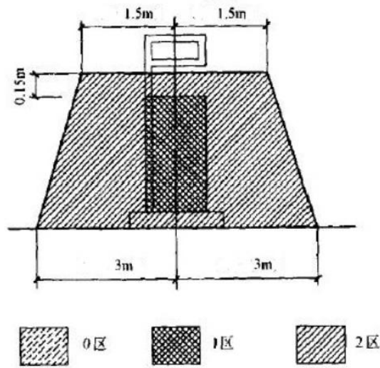
图 10-1 乙醇汽油加油机爆炸危险区域划分图
