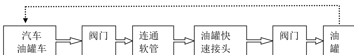
图 2-3 汽油卸油工艺流程
