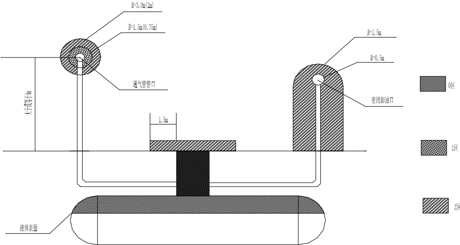
图 3-3 埋地油罐爆炸危险区域划分
