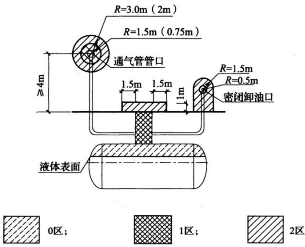
图 3-3 埋地油罐爆炸危险区域划分
