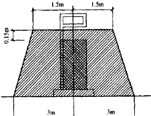
图 3.2 加油机操作危险区域划分
