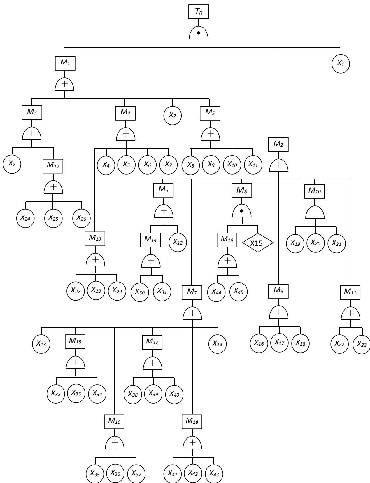
图 2-4 事故树分析
