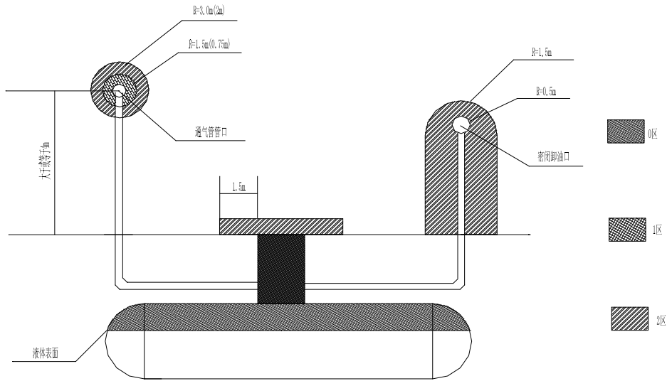
图 3-3 埋地油罐爆炸危险区域划分
