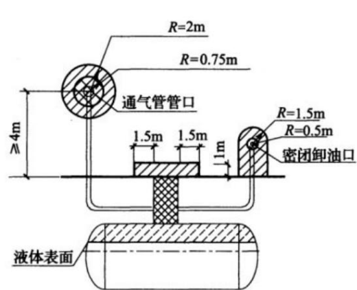
图 3-1 埋地卧式储罐爆炸危险区域划分
