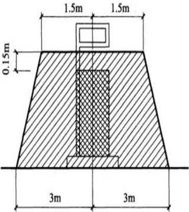
图 3-2 加油机操作危险区域划分
