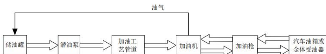
图 1-4 乙醇汽油加油工艺流程
