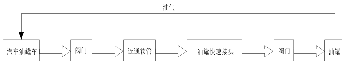
图 1-1 乙醇汽油卸油工艺流程
