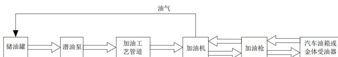
图 2-5 汽油（乙醇汽油）加油工艺框图
