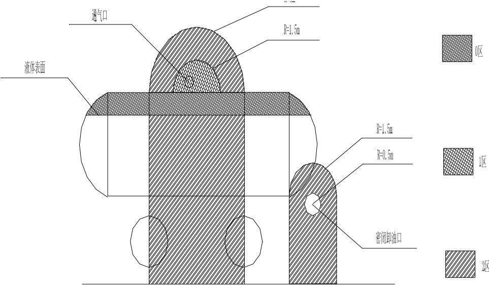
图 3-2 油罐车卸油爆炸危险区域划分
