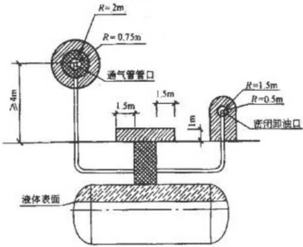
图 10-3 埋地汽油储罐爆炸危险区域划分图
