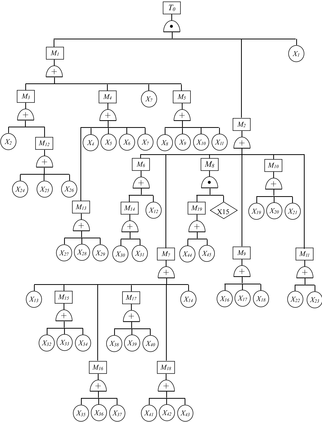
图 10-4 事故树分析
