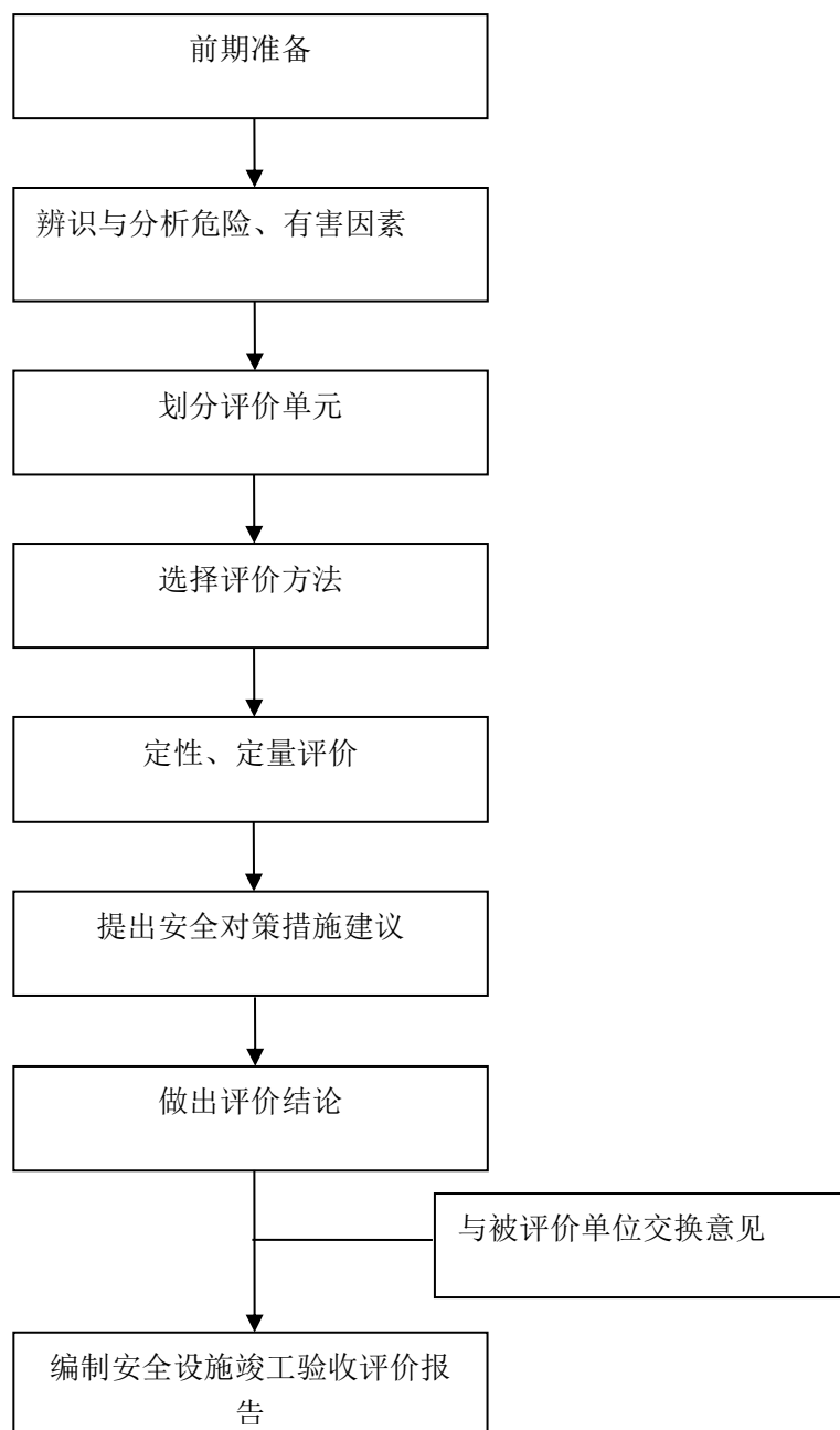
图 1-1 项目安全设施竣工验收评价的工作程序
