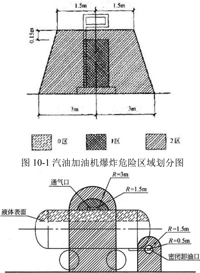
图 10-2 油罐车卸汽油爆炸危险区域划分图
