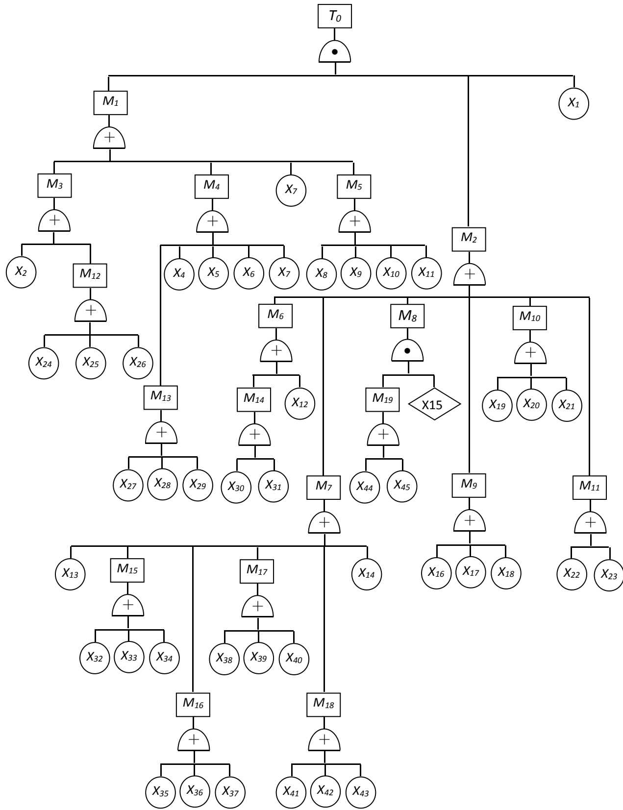
图 2-4 事故树分析
