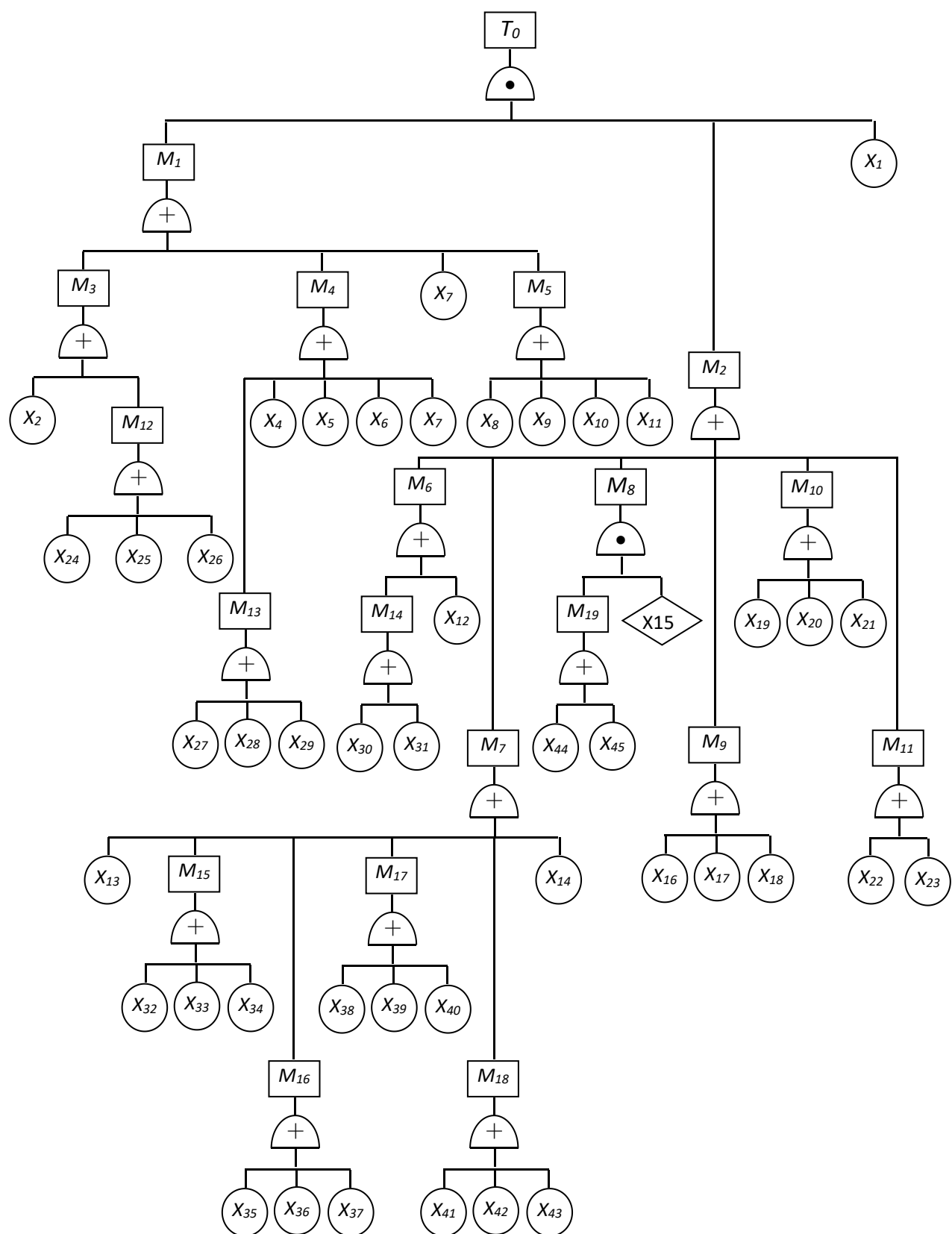
图 F2.2-1 事故树分析
