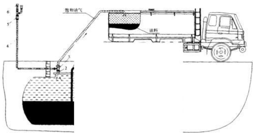
1—卸油管；2—油气回收
