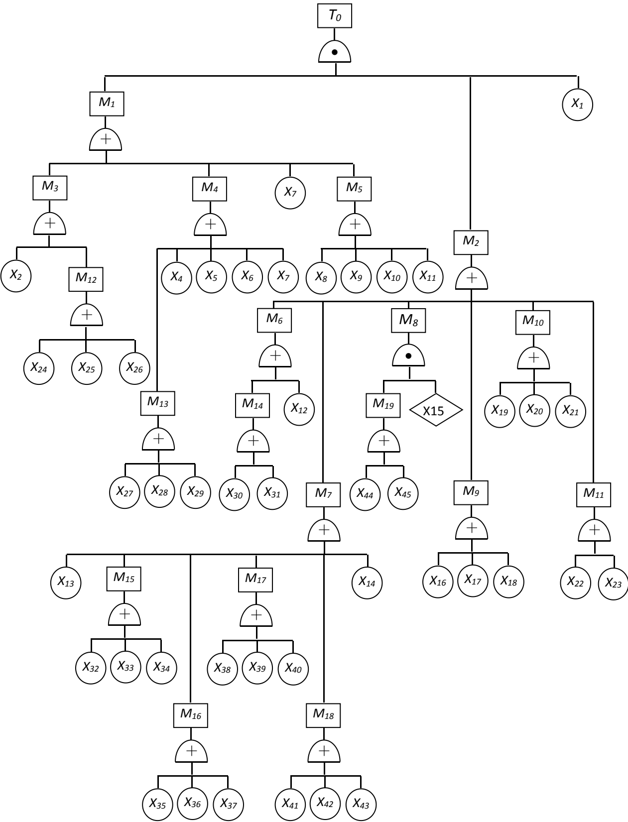
图 2-4 事故树分析
