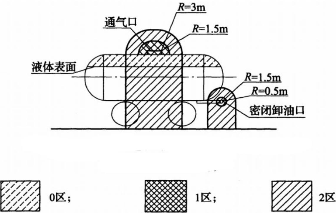
图 3-2 油罐车卸油爆炸危险区域划分
