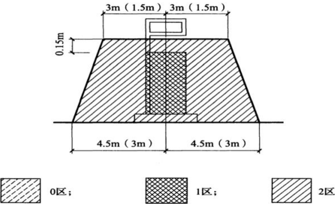
图 3-1 加油机爆炸危险区域划分
