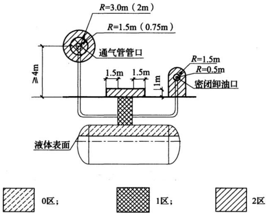
图 3-3 埋地油罐爆炸危险区域划分
