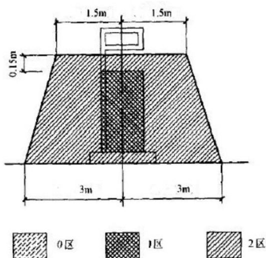
图 10-1 汽油加油机爆炸危险区域划分图
