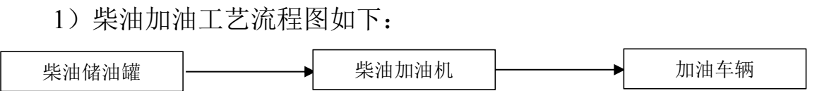
图 2-4 柴油加油工艺框图
