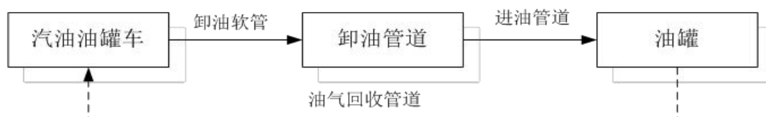
图 2-2 汽油卸油工艺框图
