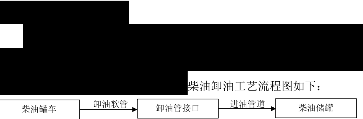
图 2-3 柴油卸油工艺框图
