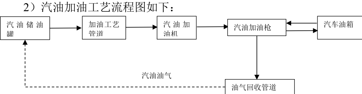
图 2-5 汽油加油工艺框图
