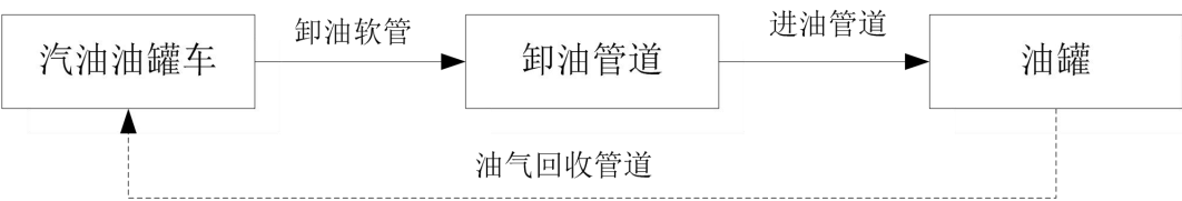
图 2-2 汽油卸油工艺框
