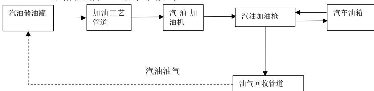
图 2-5 汽油加油工艺框
