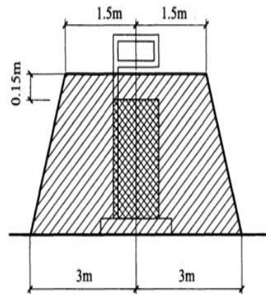
图 2-2 加油机操作危险区域划分
