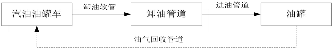
图 2-2 汽油卸油工艺框
