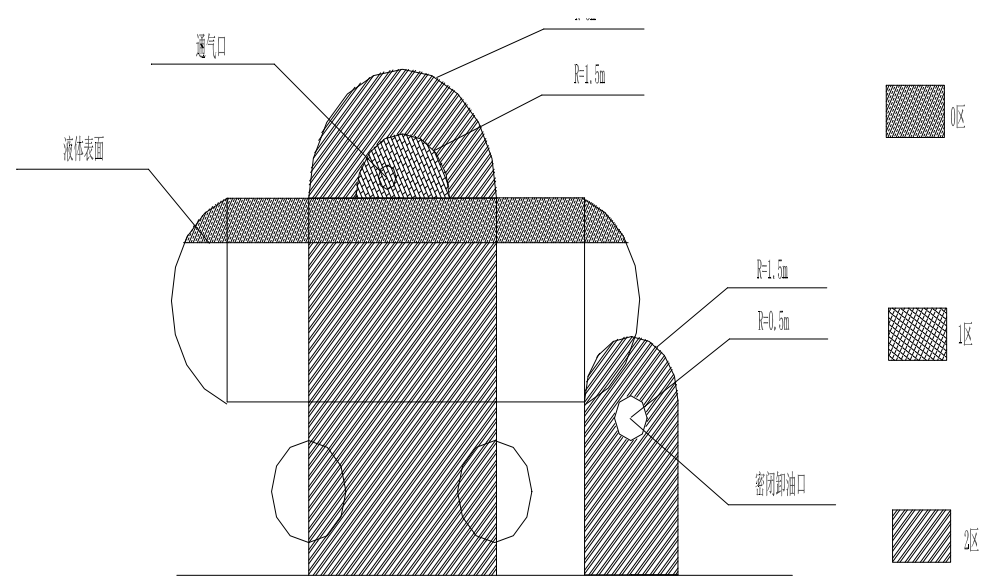
图 3-1 加油机爆炸危险区域划分
