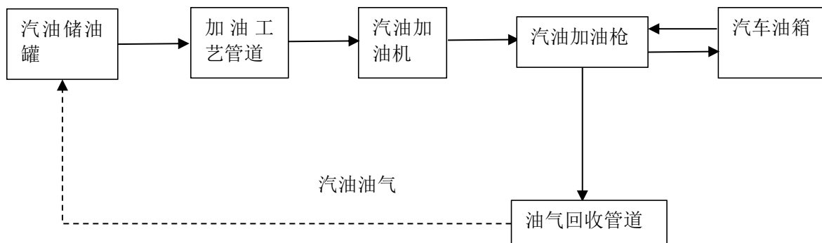
图 2-5 汽油加油工艺框图
