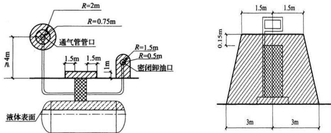
图 3-1 埋地卧式储罐爆炸危险区域划分 图 3-2 加油机操作危险区域划分
