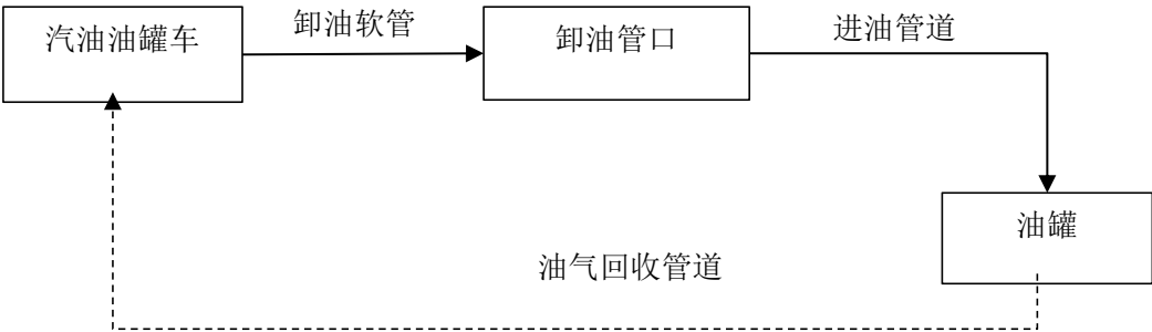
图 2-2 汽油卸油工艺框图
