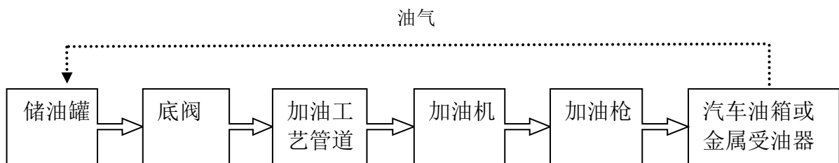
图 2-5 汽油加油工艺框图
