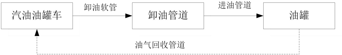
图 2-2 汽油卸油工艺框图
