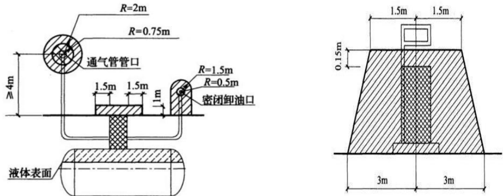
图 3-1 埋地卧式储罐爆炸危险区域划分
