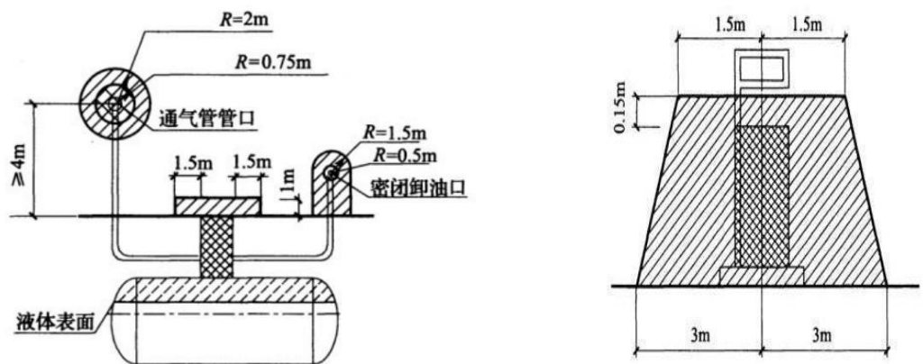
图 3-1 埋地卧式储罐爆炸危险区域划分
