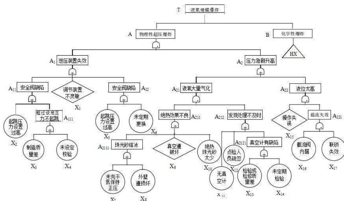
图 5.3-1 液氧储罐爆炸事故树
