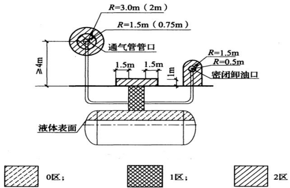
图 3-3 埋地油罐爆炸危险区域划分
