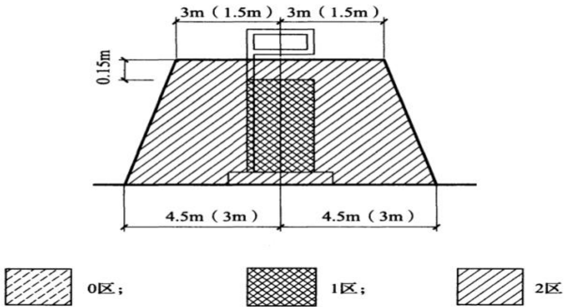
图 3-1 加油机爆炸危险区域划分
