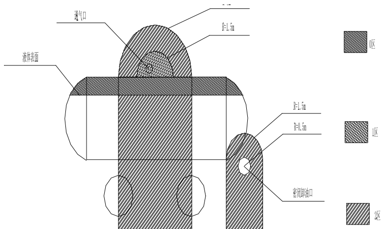
图 3-2 油罐车卸油爆炸危险
