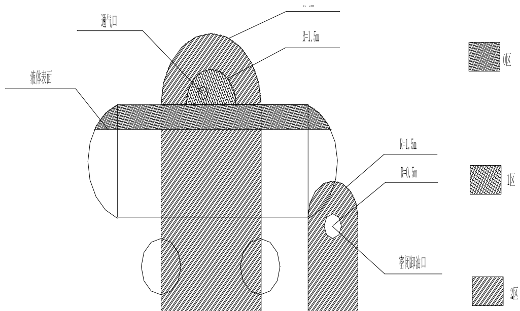
图 3-1 加油机爆炸危险区域划分
