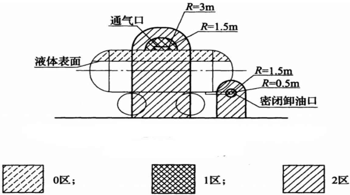
图 3-2 油罐车卸油爆炸危险区域划分
