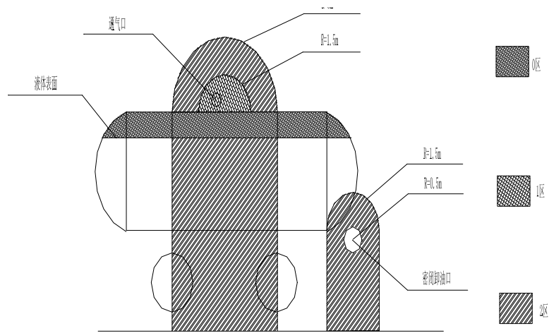
图 3-2 油罐车卸油爆炸危险区域划分
