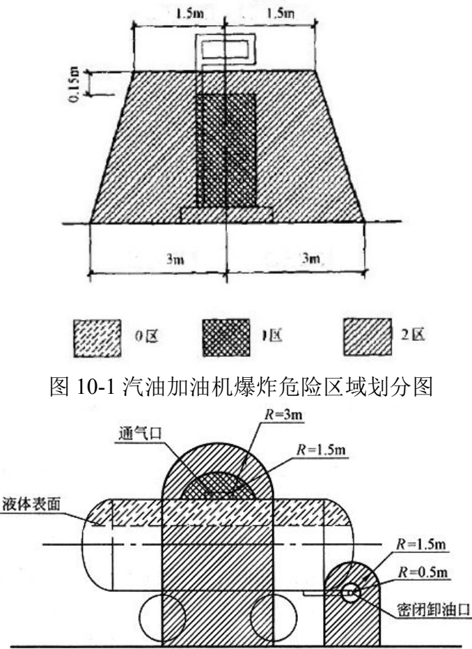
图 10-2 油罐车卸汽油爆炸危险区域划分图
