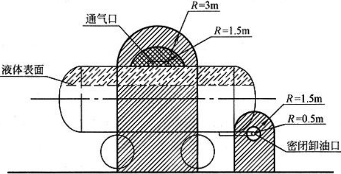
图 10-2 油罐车卸汽油爆炸危险区域划分图
