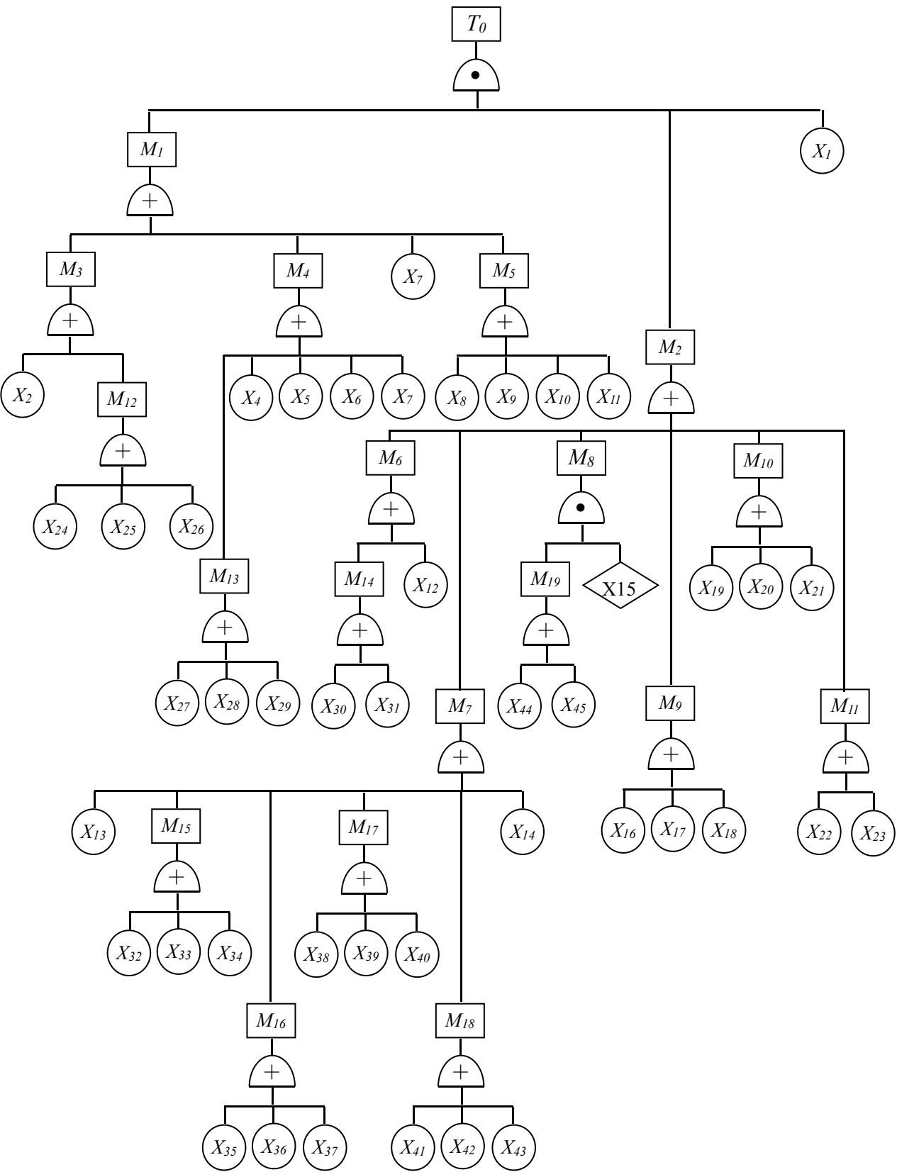
图 10-4 事故树分析
