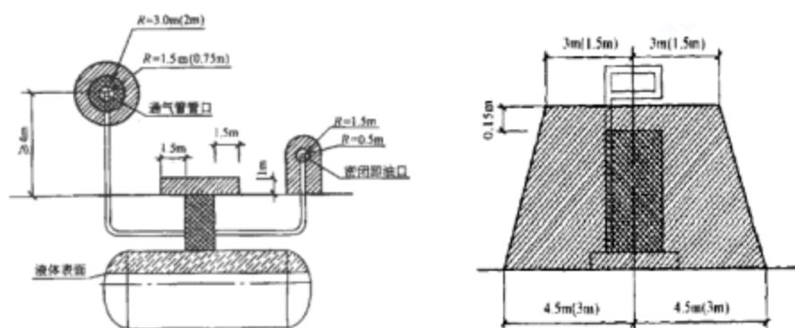
图 3.2-1 埋地卧式汽油储罐爆炸危险区域划分图
